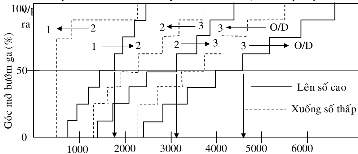
Hình 4.6: Sơ đồ chuyển số S - 2: vị trí D, chế độ tải nặng.
