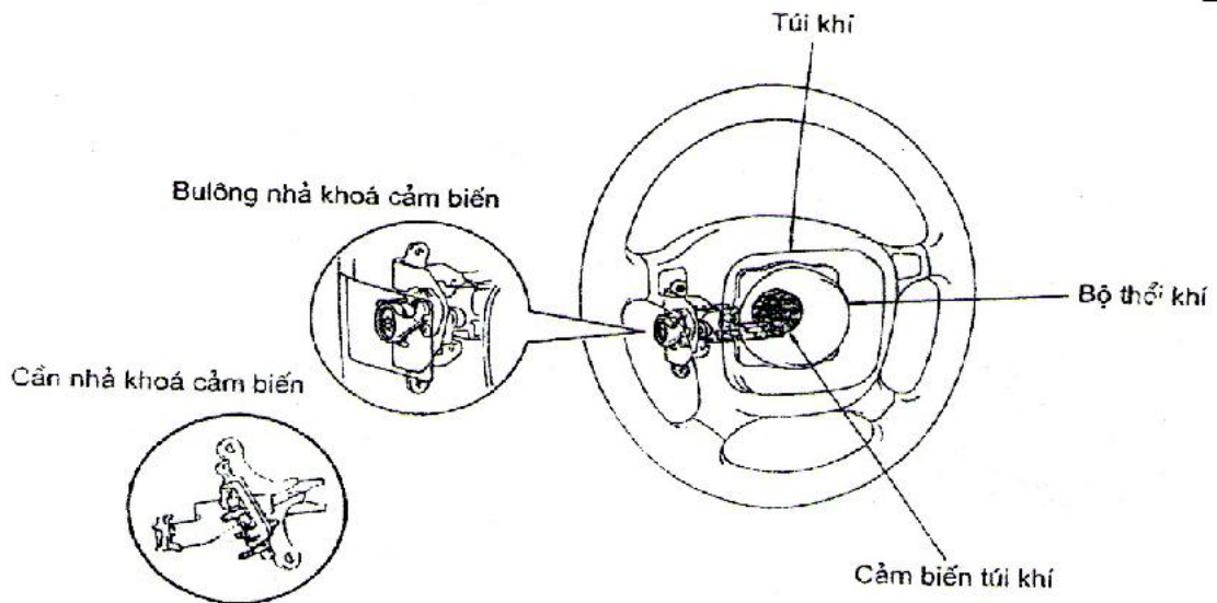
Hình 6.23: Sơ đồ bố trí các chi tiết
