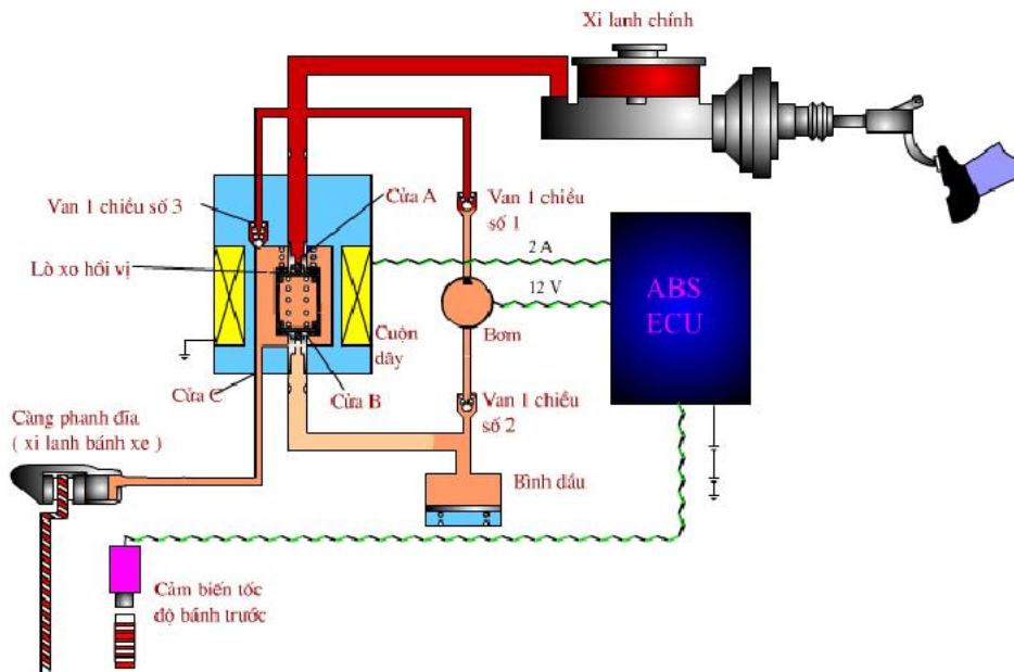
Hình 5.30: Pha giữ áp.
