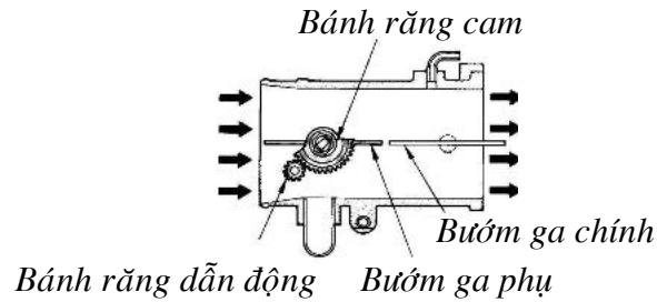
Hình 5.41: Vị trí bướm ga phụ mở hoàn toàn
