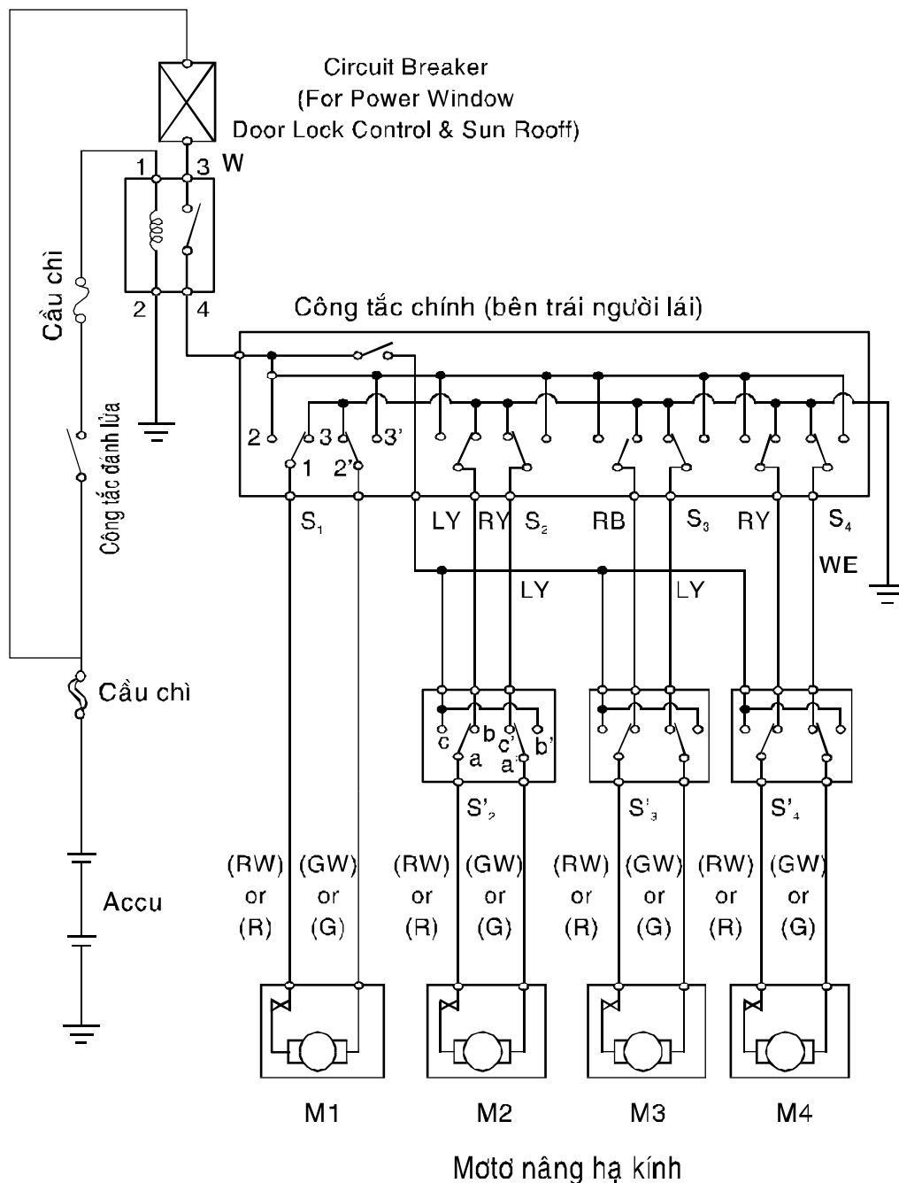
Hình 3.23: Sơ đồ mạch điện nâng hạ cửa trên xe TOYOTA CRESSIDA.
