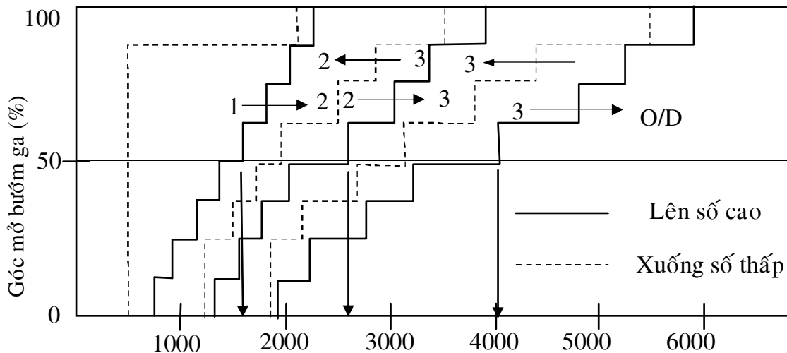
Hình 4.5: Sơ đồ chuyển số S-1: vị trí D, chế độ bình thường.
