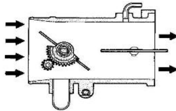
Hình 5.42: Vị trí bướm ga phụ mở 50%
