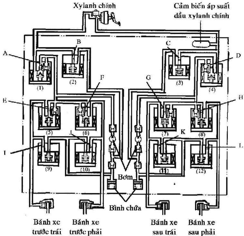
Hình 5-36: Sơ đồ hoạt động của ABS với EBD vàBAS.
