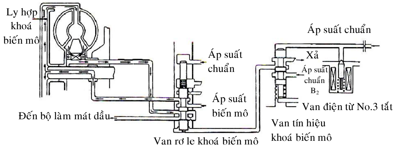
Hình 4.25: Ly hợp khoá biến mô mở.
