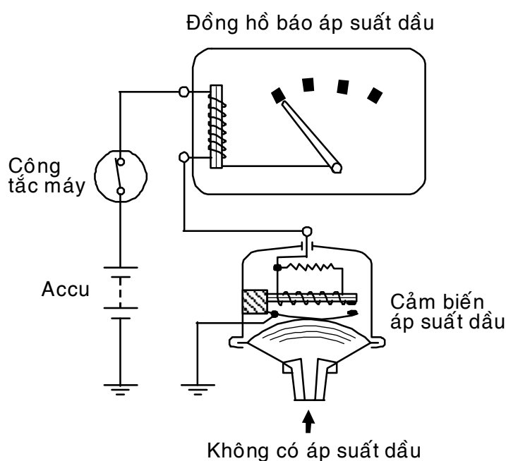
Hình 1.7 Hoạt động của đồng hồ nhiệt điện khi áp suất nhớt thấp/nhỏ.
