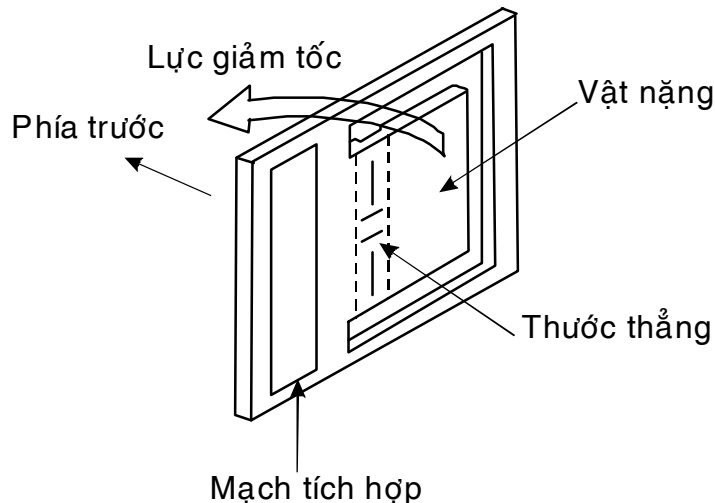
Hình 6.9: Cảm biến túi khí trung tâm loại bán dẫn
