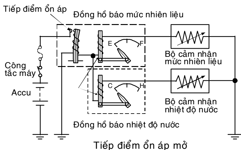
Hình 1.12 Hoạt động của đồng hồ kiểu điện trở lưỡng kim khi tiếp điểm ổn áp đóng/mở.
