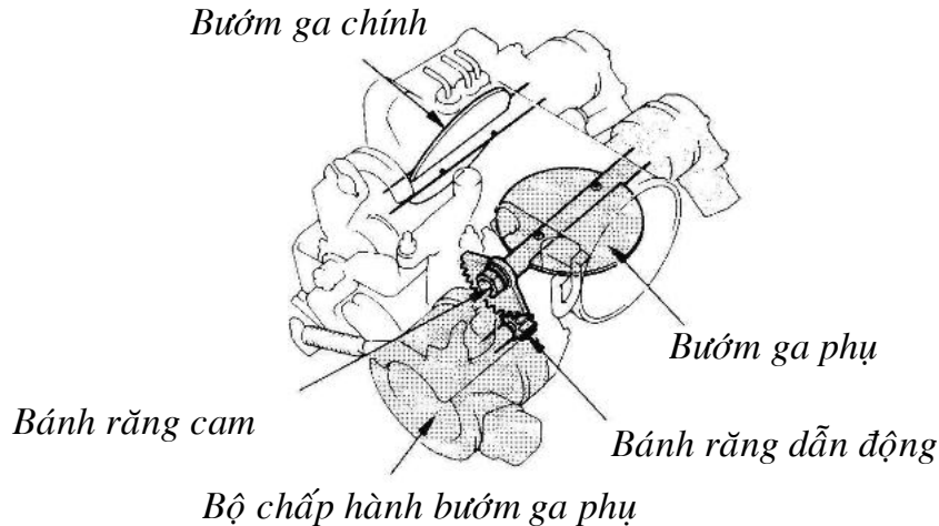
Hình 5.39: Vị trí bộ chấp hành bướm ga phụ
