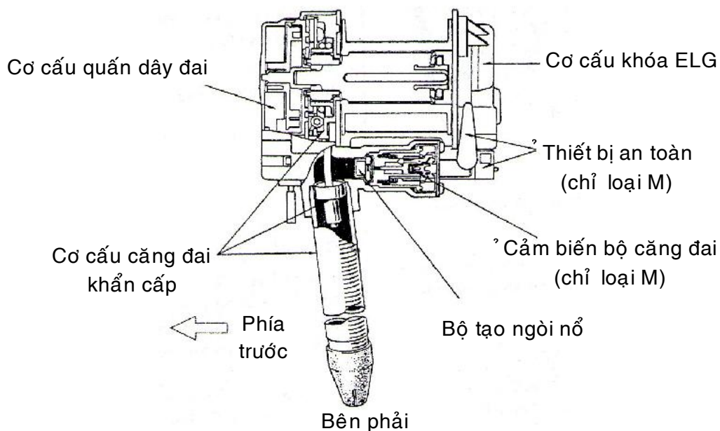
Hình 6.4: Kết cấu hệ thống điều khiển đai an toàn
