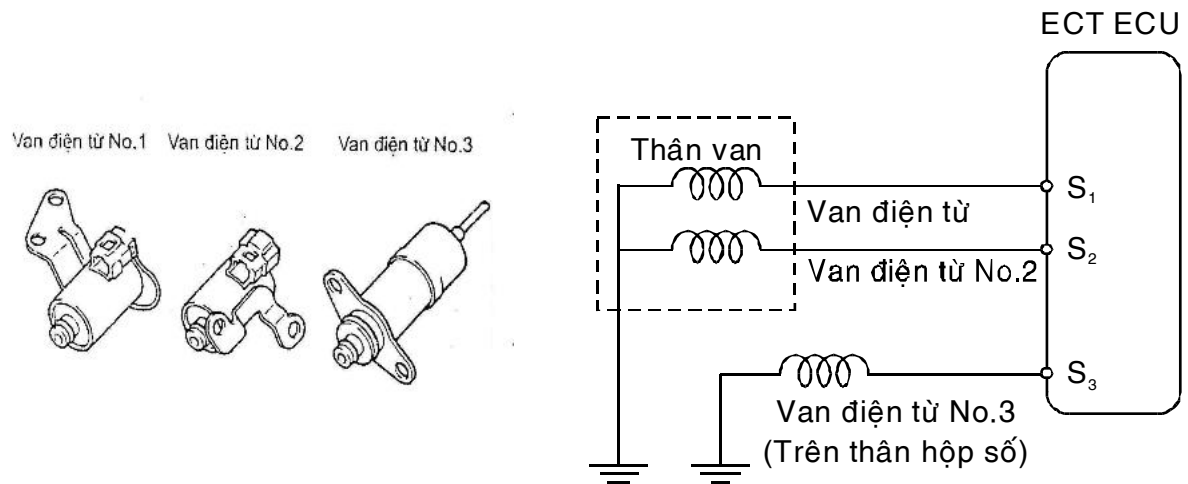
Hình 4.45 : Các van điện.
