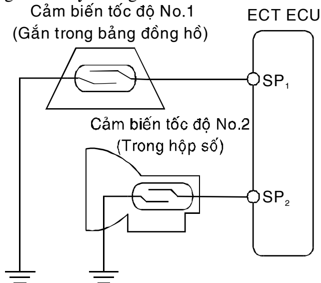
Hình 4.38: Sơ đồ các cảm biến tốc độ trong hệ thống.
