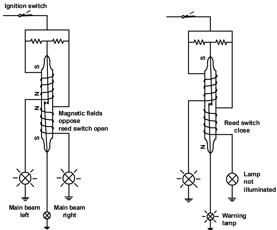
Hình 2.36: Sơ đồ nguyên lý của mạch báo đứt bóng dùng công tắc lưới gà
