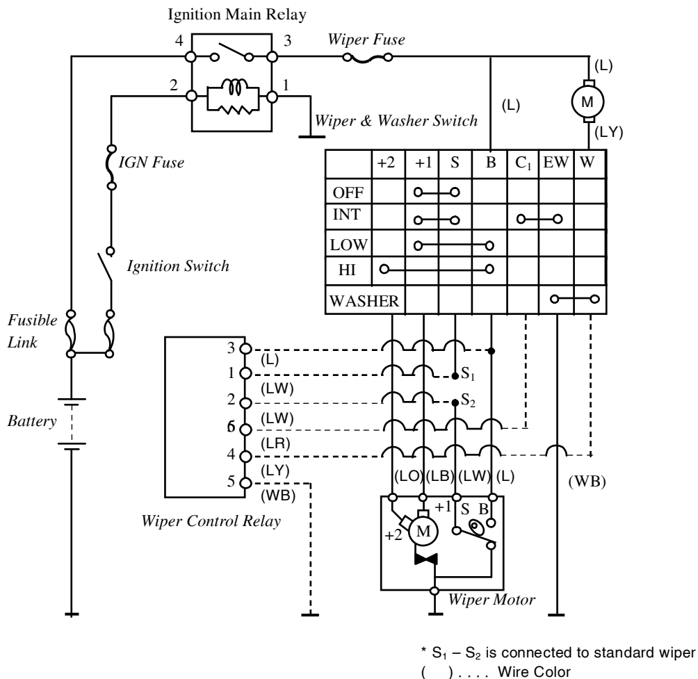
Hình 3.13: Sơ đồ mạch điện gạt và phun nước kính trước xe TOYOTA CRESSIDA
