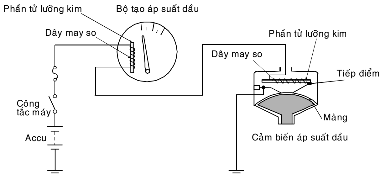
Hình 1.5 Sơ đồ cấu tạo đồng hồ áp suất nhớt.
