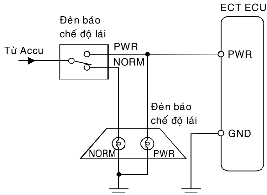
Hình 4.30: Công tắc chọn chế độ hoạt động.
