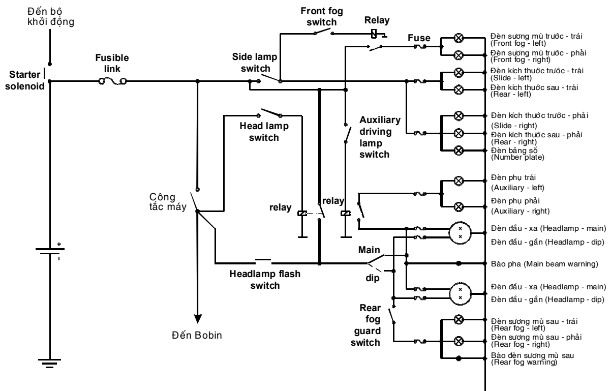
Hình 2.1: Sơ đồ mạch điện chiếu sáng trên ô tô
