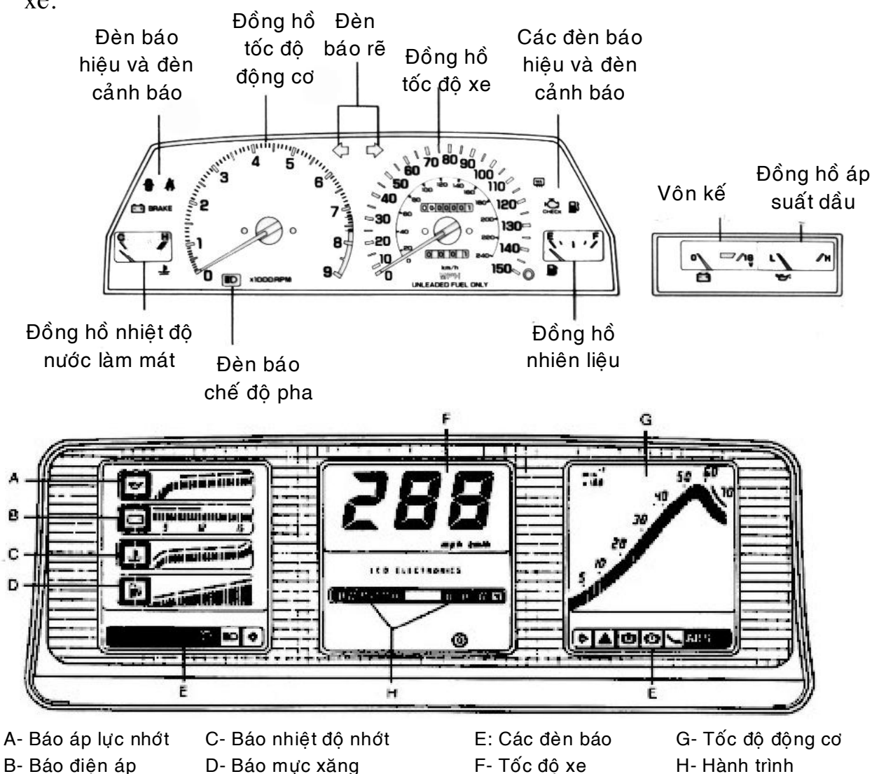
Hình 1.1 Cấu tạo bảng tableau loại thường và loại hiện số.
