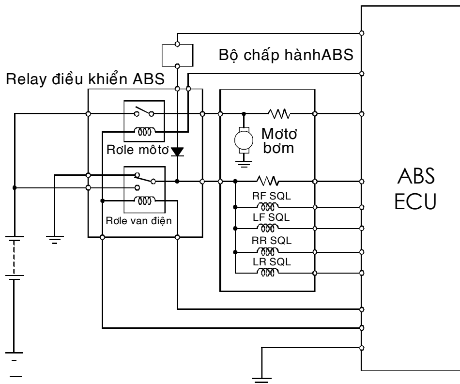
Hình 5.33: Sơ đồ điều khiển các relay
