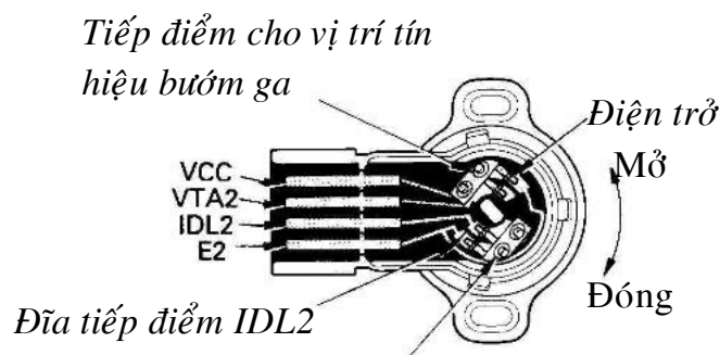
Hình 5.44: Cấu tạo cảm biến vị trí bướm ga
