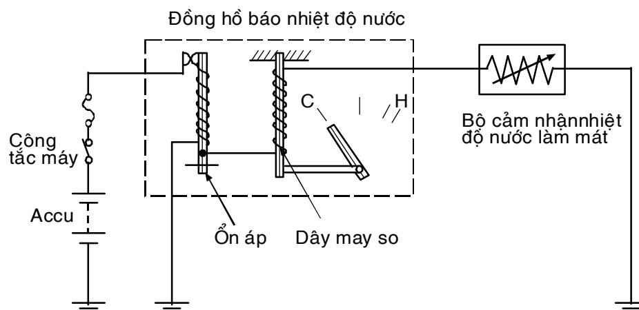
Hình 1.19 Hoạt động của đồng hồ nước làm mát.
