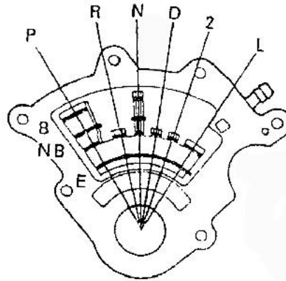
Hình 4.32: Công tắc khởi động số trung gian.
