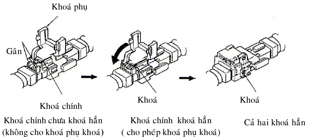
Hình 6.18: Cơ cấu khoá giấc kép
