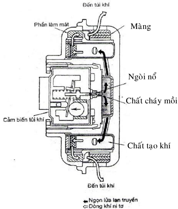
Hình 6.28: Mô tả hoạt động của bộ thổi khí và túi khí
