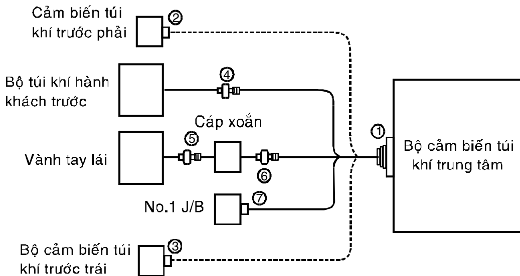
Hình 6.14: Vị trí các giắc nối
