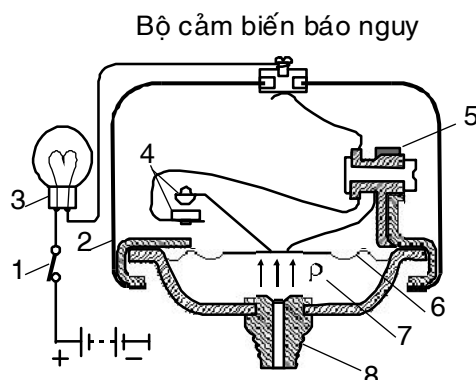
Hình 1.28 Cơ cấu báo nguy áp suất dầu bôi trơn động cơ.
