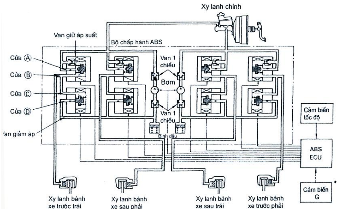
Hình 5.32: Sơ đồ bộ chấp hành thủy lực loại 8 van điện 2 vị trí.
