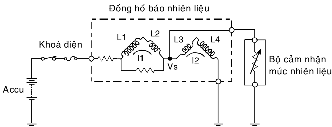
Hình 1.13 Đồng hồ nhiên liệu kiểu cuộn dây chữ thập.
