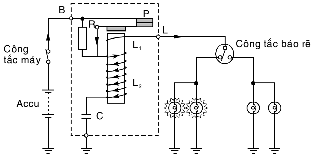
Hình 2.23: Tiếp điểm đóng (đèn báo rẽ sáng)
