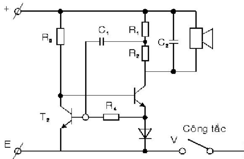
Hình 2.17: Sơ đồ mạch chuông nhạc
