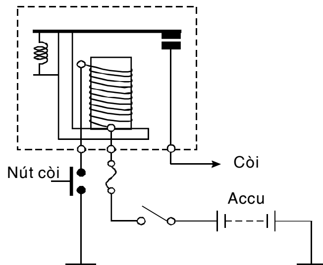
Hình 2.15: Rơle còi
