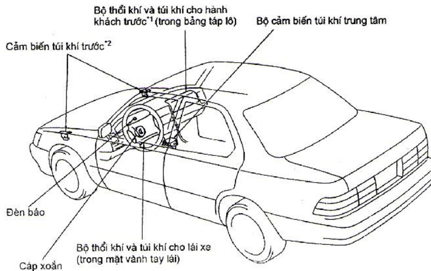
Hình 6.5: Sơ đồ bố trí các chi tiết
