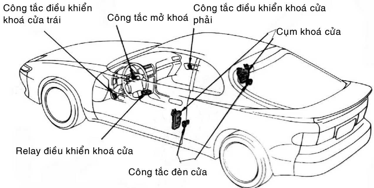
Hình 3.15: Các chi tiết trên hệ thống khoá cửa.
