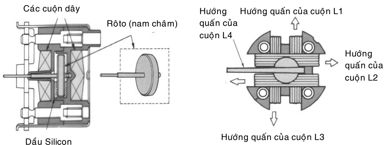
Hình 1.14 Cấu tạo đồng hồ nhiên liệu kiểu cuộn dây chữ thập.
