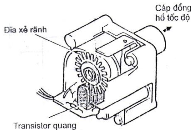
Hình 7.9: Cảm biến tốc độ loại quang
